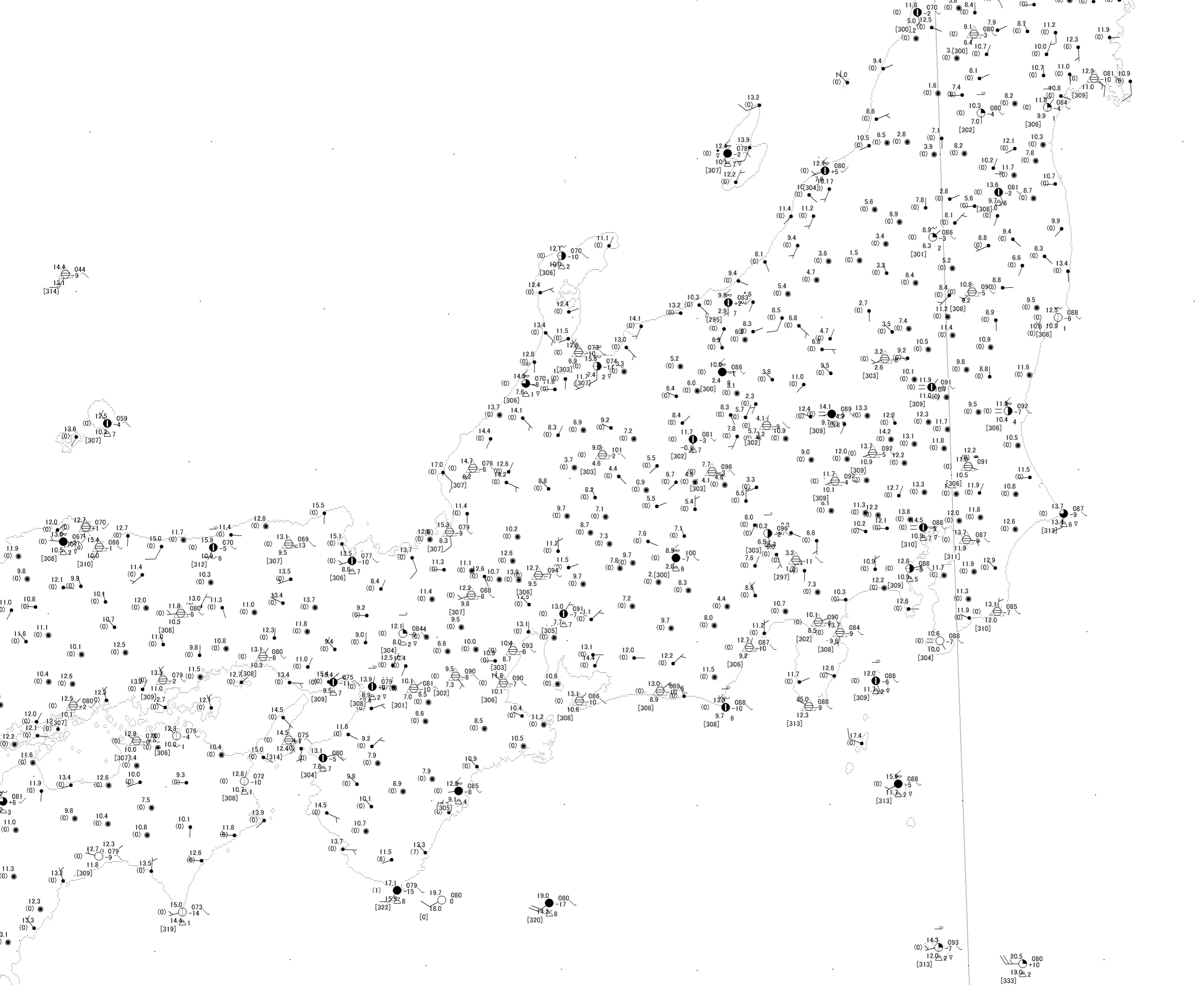
291800UTC APR.2006 アメダスデータ(今市) 本図のデータは気象庁公式サイトの 観測データによっています 地図データはアメリカ地質調査所の 標高データによっています [気象予報士会埼玉支部]
