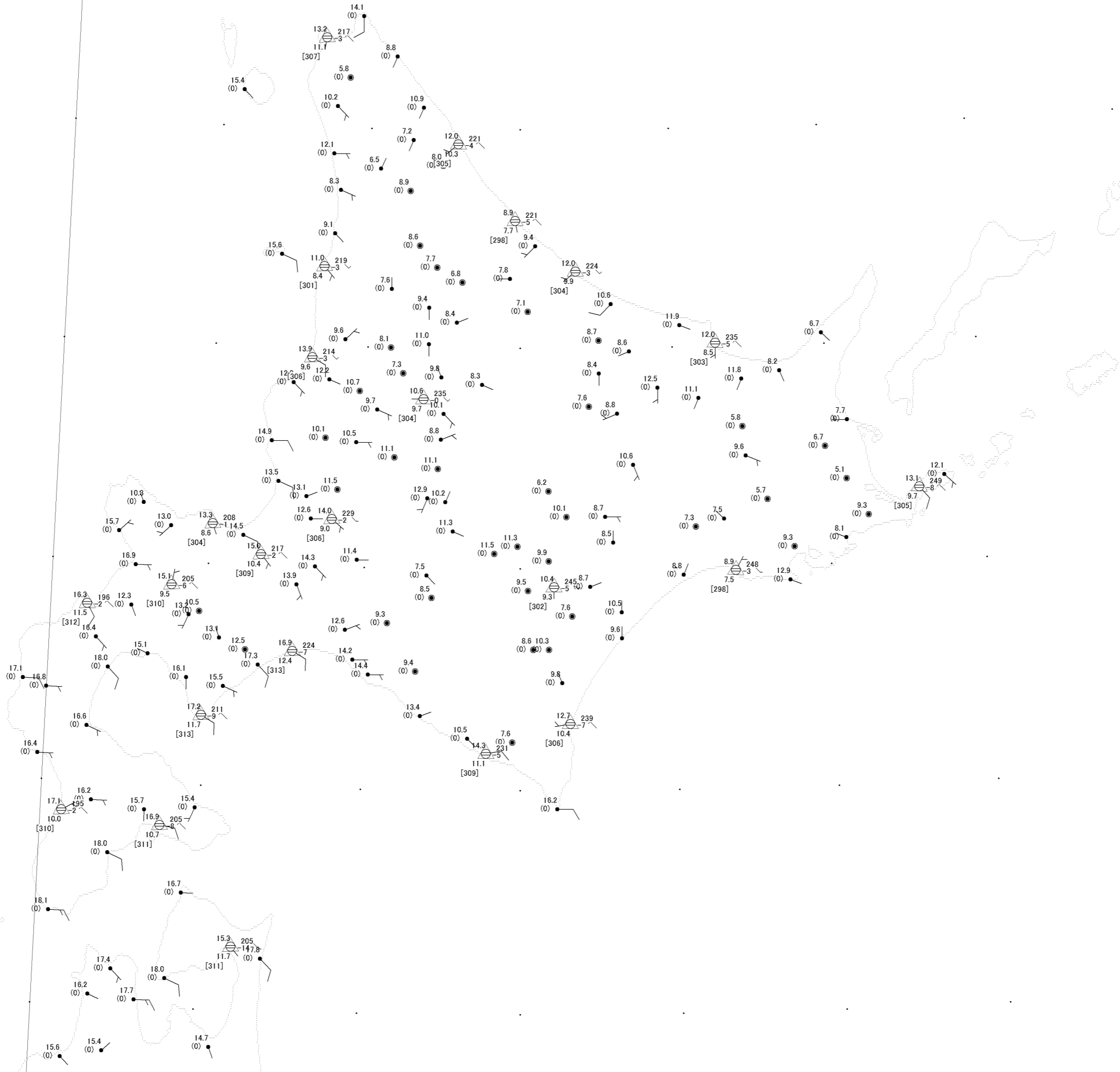
261700UTC SEP.2006 アメダスデータ(北海道) 本図のデータは気象庁公式サイト の観測データによっています 地図データはアメリカ地質調査所 の標高データによっています [気象予報士会埼玉支部]
