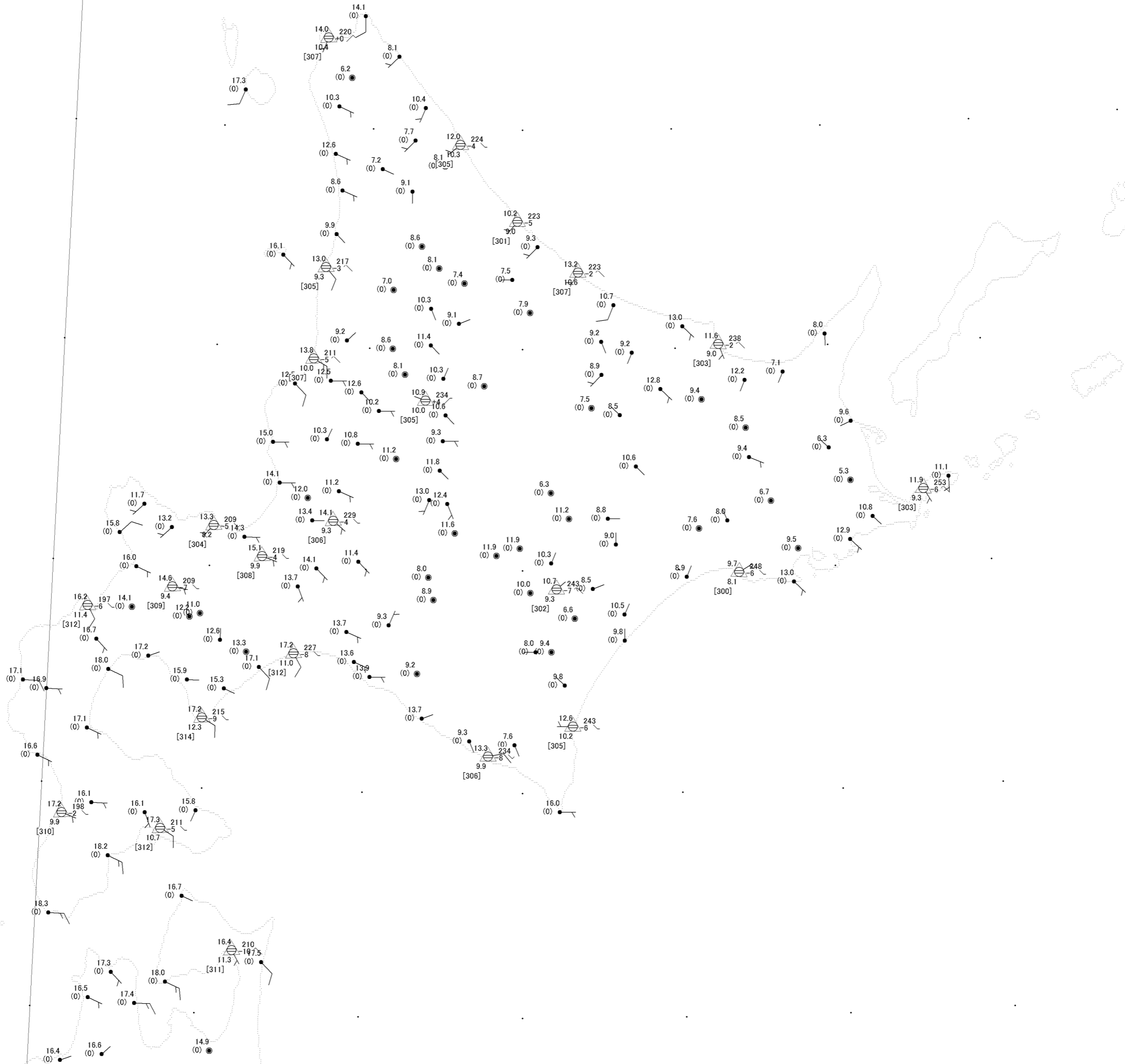
261600UTC SEP.2006 アメダスデータ(北海道) 本図のデータは気象庁公式サイト の観測データによっています 地図データはアメリカ地質調査所 の標高データによっています [気象予報士会埼玉支部]
