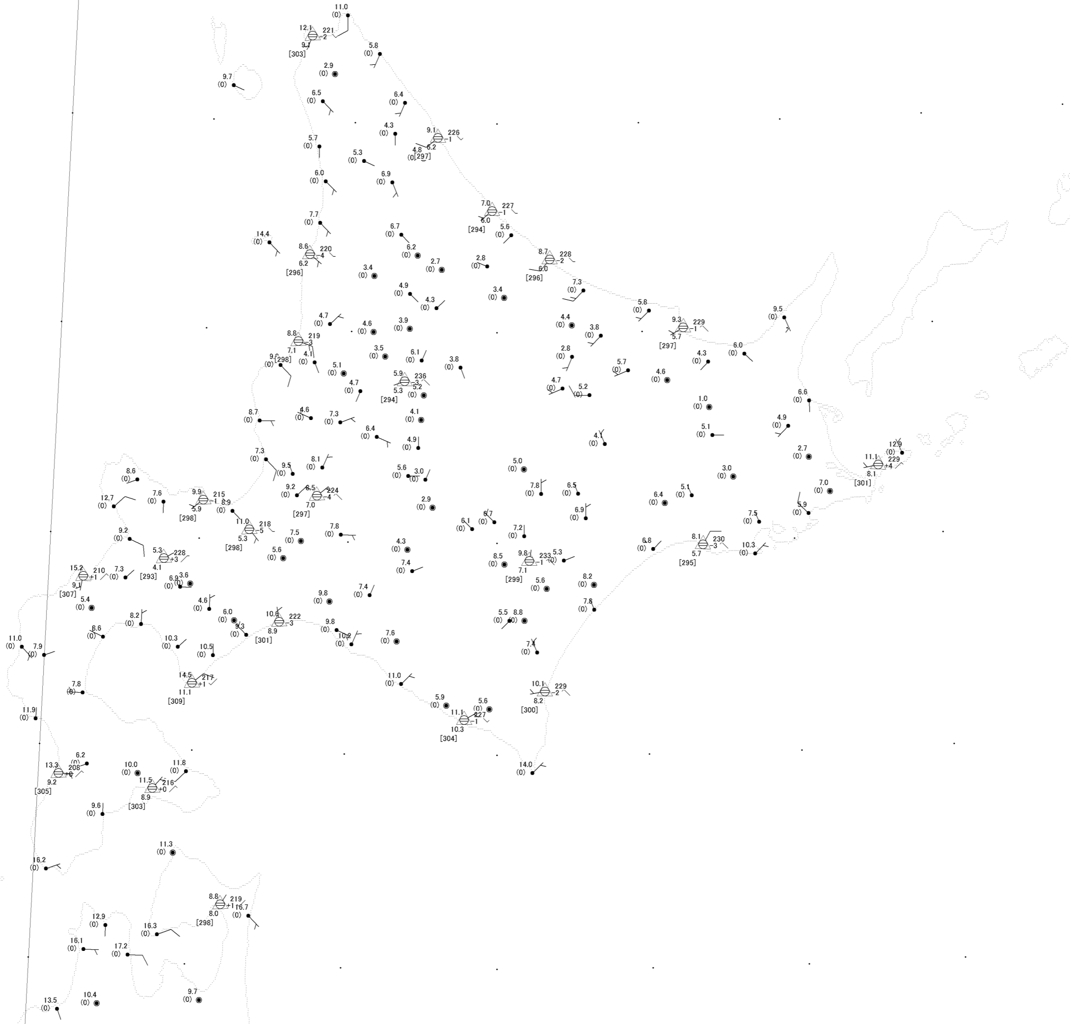
251700UTC SEP.2006 アメダスデータ(北海道) 本図のデータは気象庁公式サイトの 観測データによっています 地図データはアメリカ地質調査所の 標高データによっています [気象予報士会埼玉支部]
