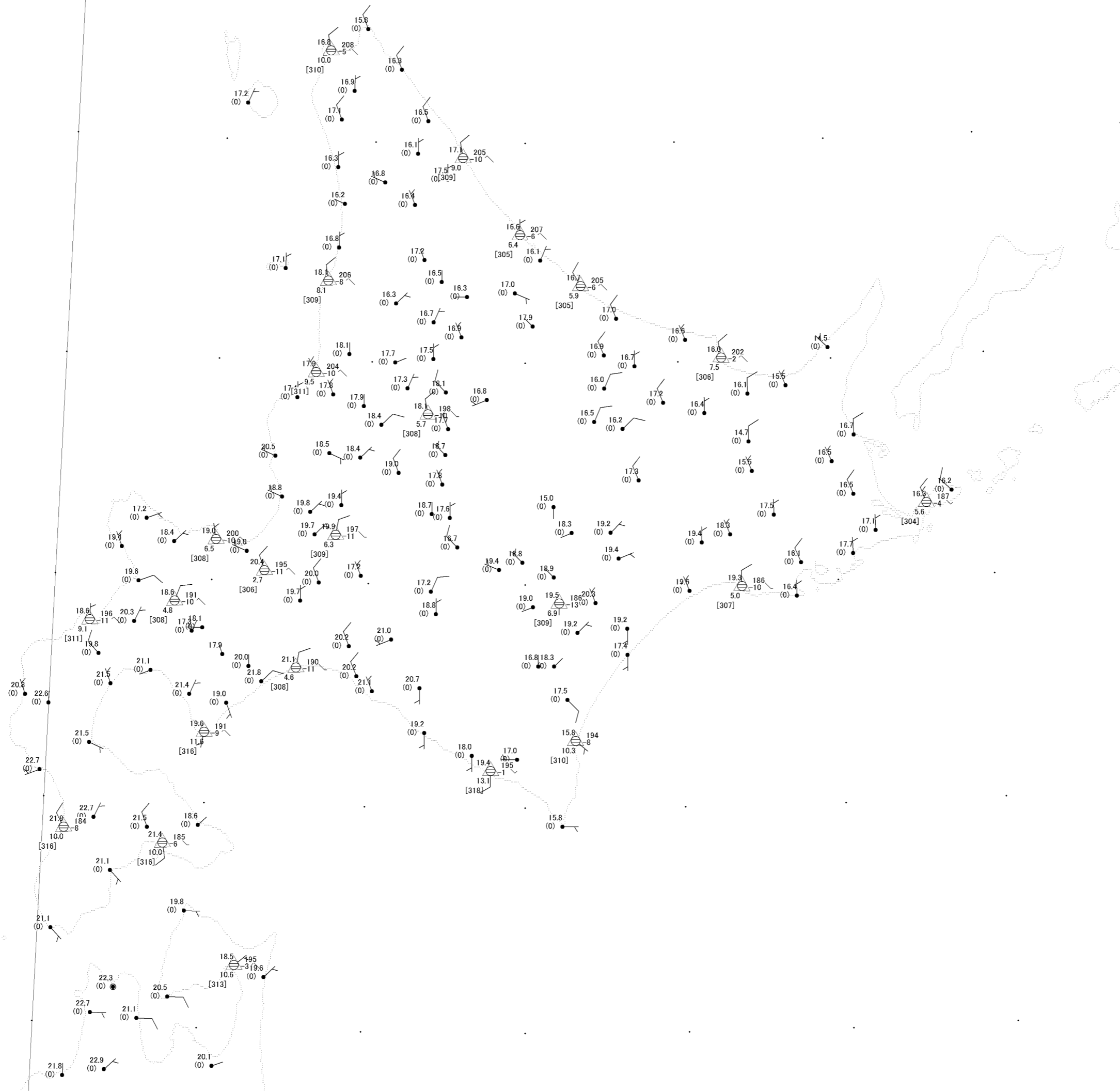
250500UTC SEP.2006 アメダスデータ(北海道) 本図のデータは気象庁公式サイトの 観測データによっています 地図データはアメリカ地質調査所の 標高データによっています [気象予報士会埼玉支部]
