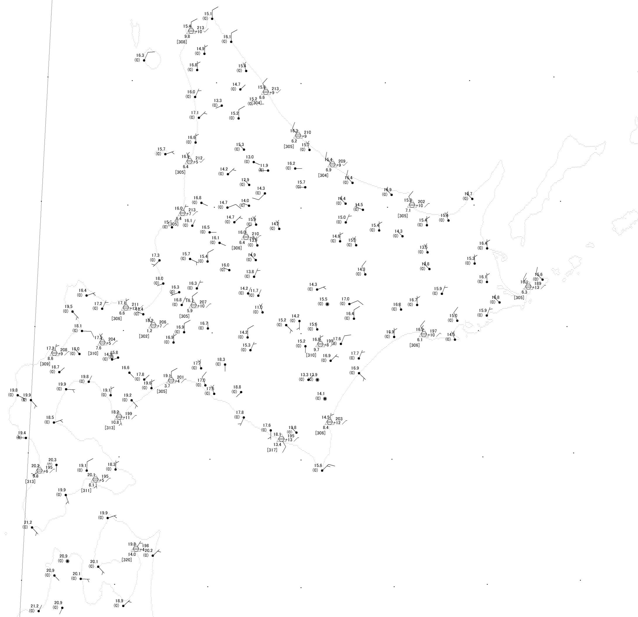
250100UTC SEP.2006 アメダスデータ(北海道) 本図のデータは気象庁公式サイトの観測データによっています 地図データはアメリカ地質調査所の標高データによっています [気象予報士会埼玉支部]
