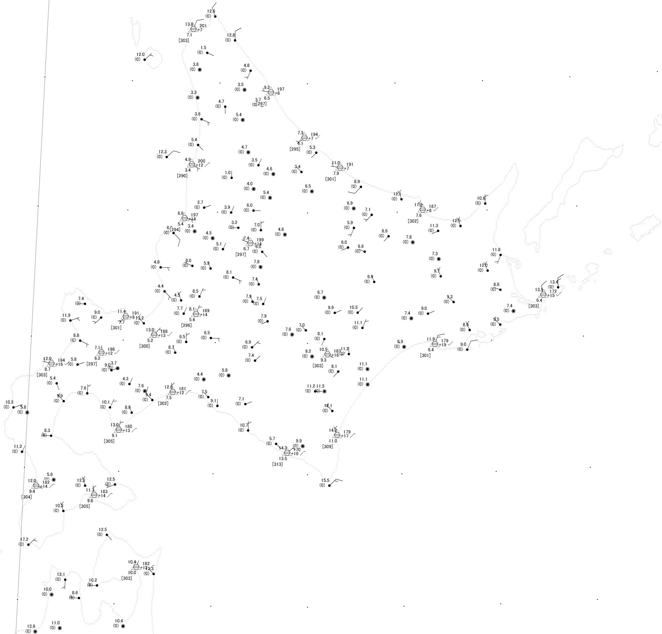
242000UTC SEP.2006 アメダスデータ(北海道) 本図のデータは気象庁公式サイト の観測データによっています 地図データはアメリカ地質調査所 の標高データによっています [気象予報士会埼玉支部]
