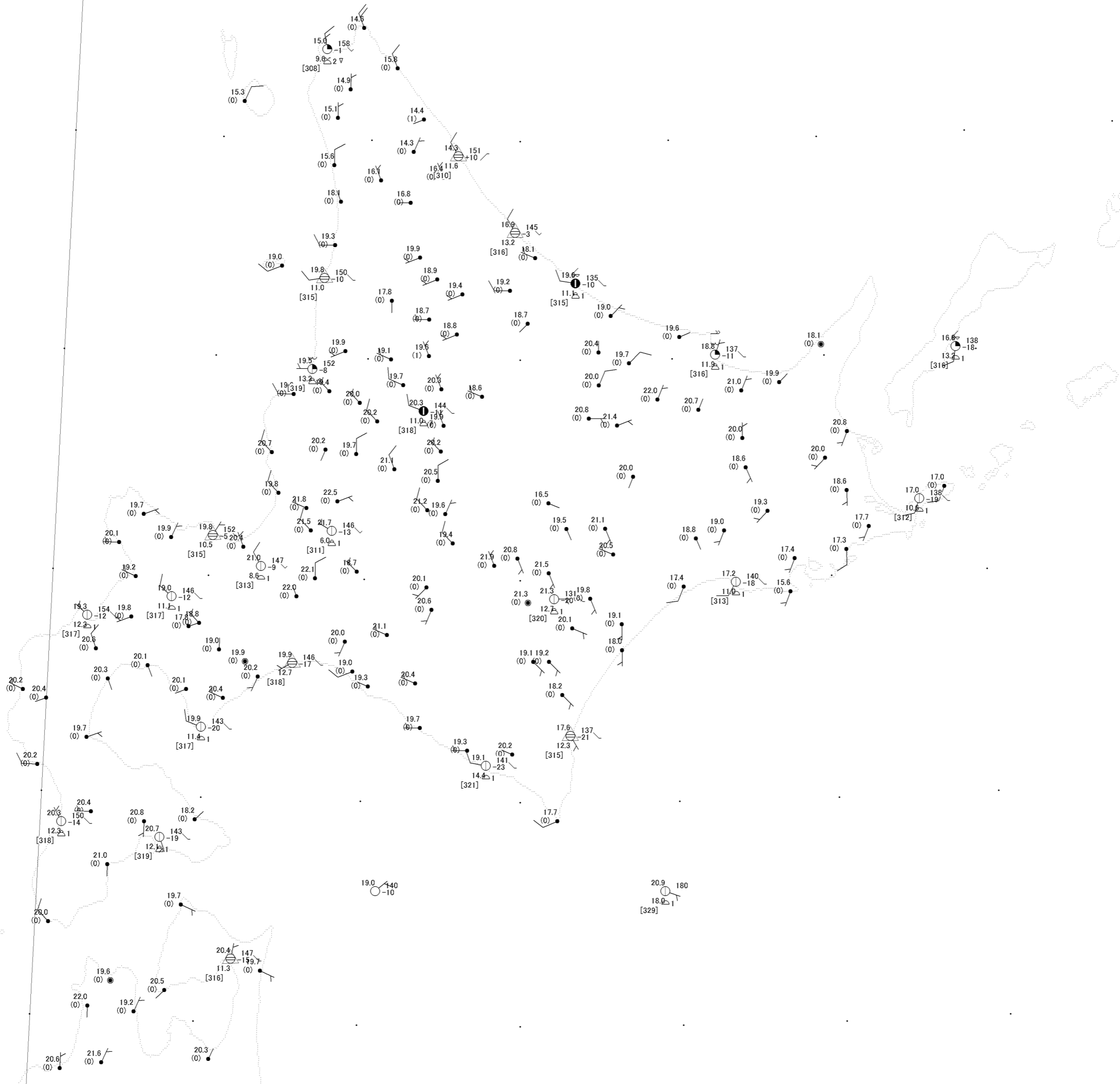
240600UTC SEP.2006 アメダスデータ(北海道) 本図のデータは気象庁公式サイト の観測データによっています 地図データはアメリカ地質調査所 の標高データによっています [気象予報士会埼玉支部]
