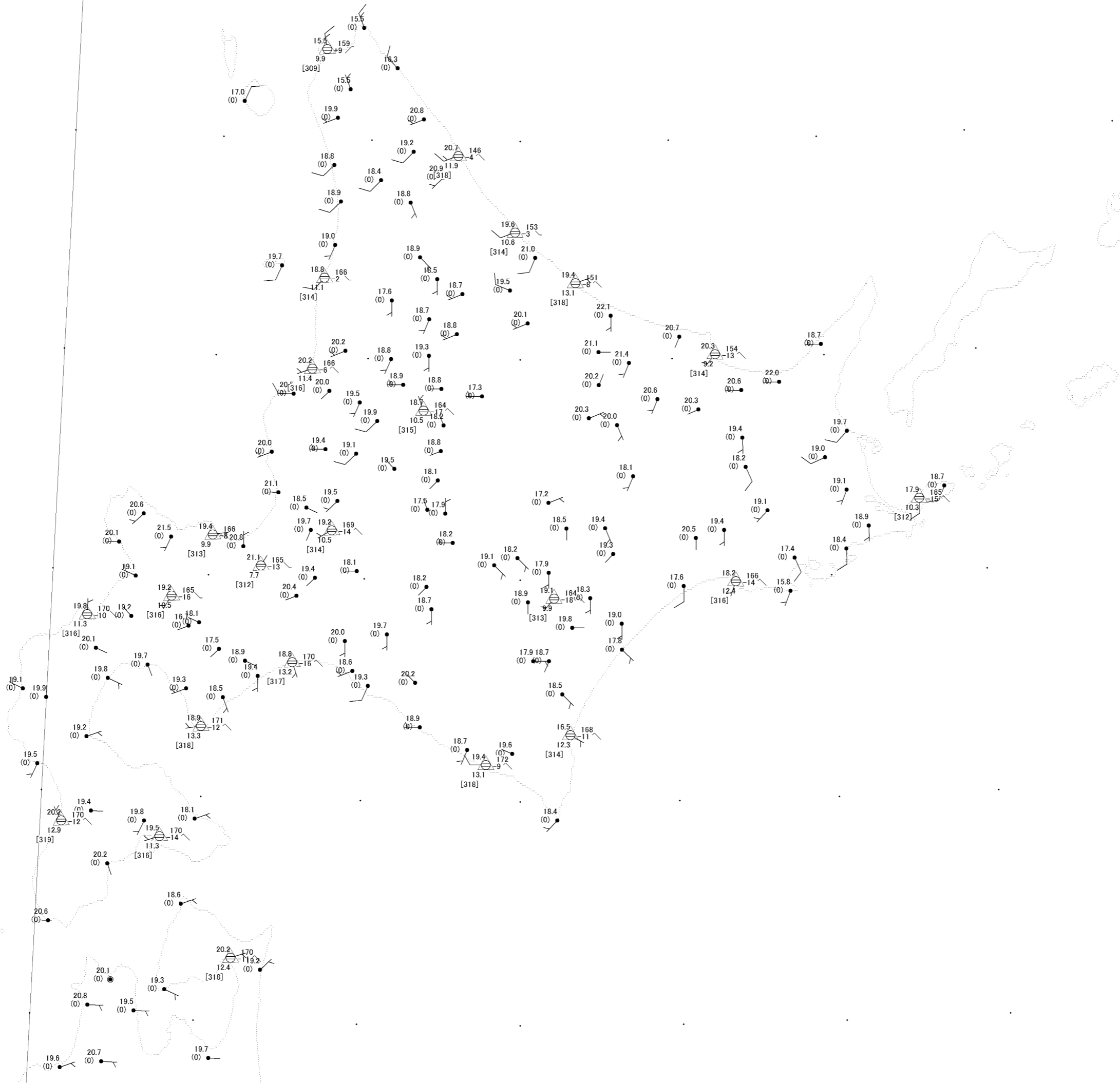
240200UTC SEP.2006 アメダスデータ(北海道) 本図のデータは気象庁公式サイト の観測データによっています 地図データはアメリカ地質調査所 の標高データによっています [気象予報士会埼玉支部]
