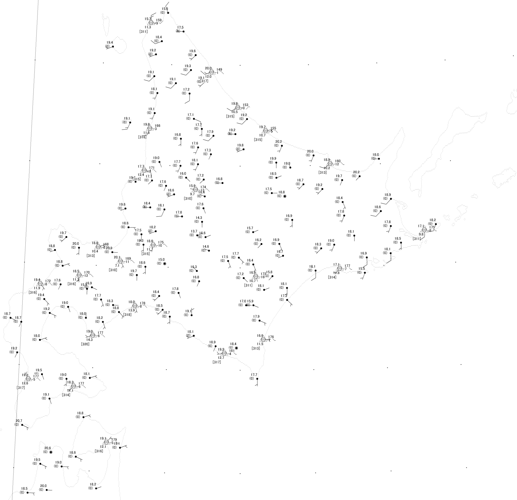
240100UTC SEP.2006 アメダスデータ(北海道) 本図のデータは気象庁公式サイトの 観測データによっています 地図データはアメリカ地質調査所の 標高データによっています [気象予報士会埼玉支部]
