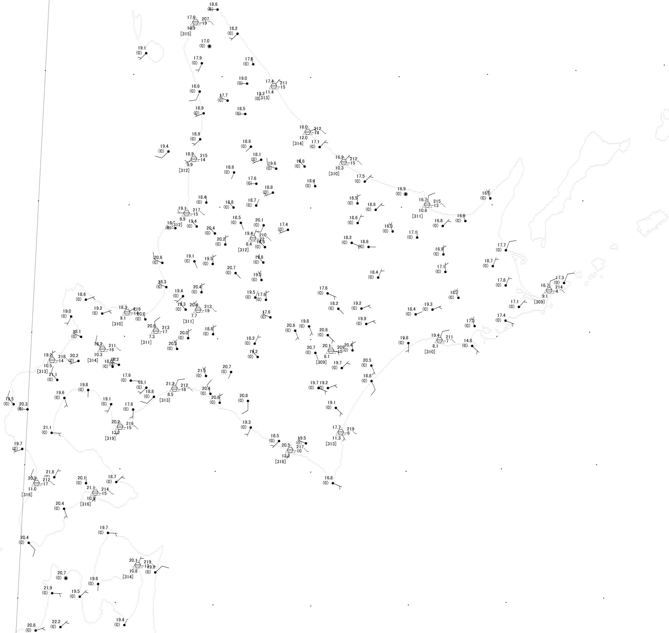
230400UTC SEP.2006 アメダスデータ(北海道) 本図のデータは気象庁公式サイトの 観測データによっています 地図データはアメリカ地質調査所の 標高データによっています [気象予報士会埼玉支部]
